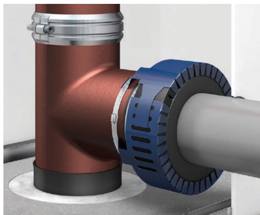
CurafLAM® Konfix Pro - Brandabschottung von Mischinstallationen
