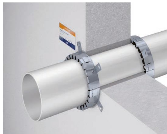
CurafLAM® Segment SM Pro im Massivwand-Einbau
