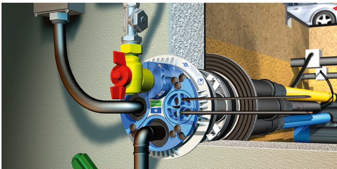
Quadro-Sicura® Nova führt alle Versorgungsleitungen gebündelt ins Haus
